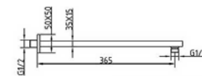
BPO02CR Retangular à parede 35x15 c/ 365mm Braço retangular en pared 35x15 c/ 365mm
