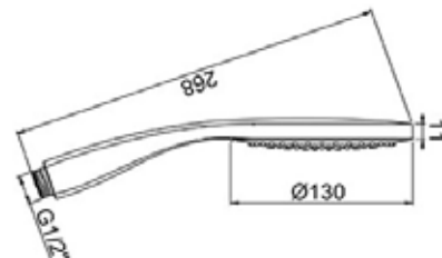
CHMECO130 Chuveiro cromado Ø100 ECOAIR Ducha de mano Ø100 ECOAIR
