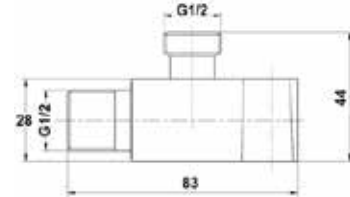
SPLQ01 Suporte chuveiro quadrado c/ saída de água cromado Soporte ducha cuadrado con conexión
